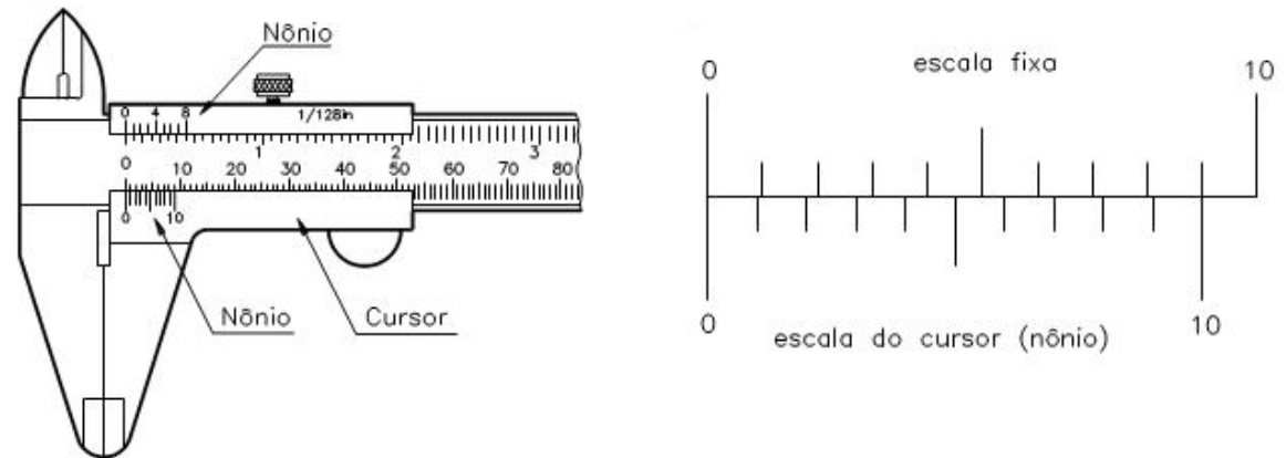
Figura 7 – Paquímetro e detalhe do nônio
