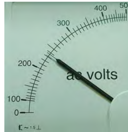
Figura 3 – Leitura de uma grandeza em um instrumento de medição analógico
